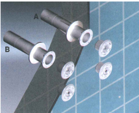
Pormenor instalação Passamuros Piscina betão
